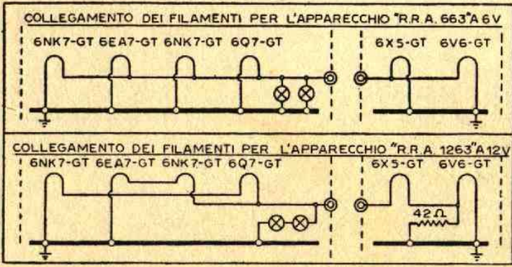
Lo schema elettrico dell'Autovox RRA 663 - RRA 1263.
